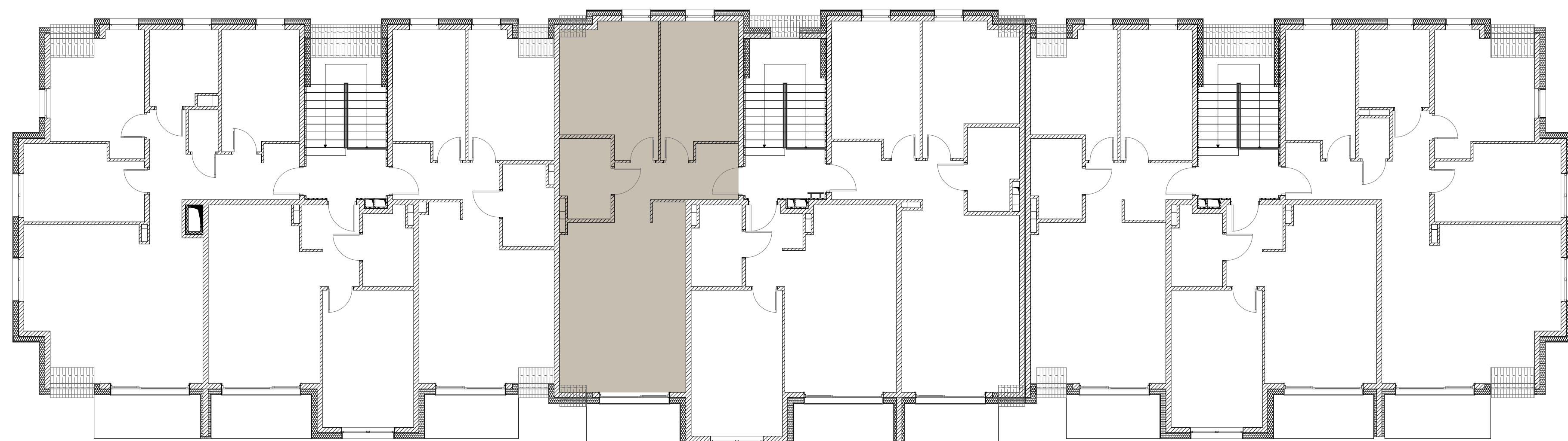
SCHEMAT KONDYGNACJI
